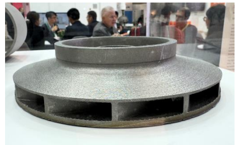
サポート材不要の造形事例 金属製ポンプ羽根車
